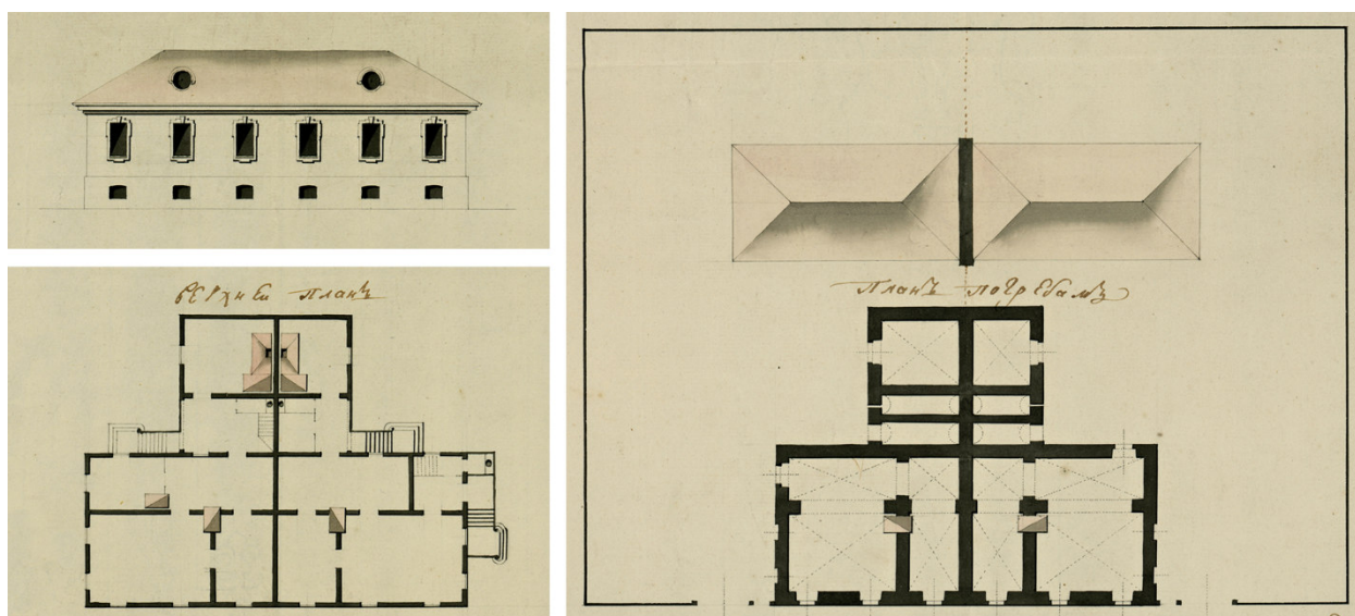
Рис. 3. Чертеж дома мазанки. Архитектор Андрей Меньшой. Ноябрь 1767 года (отредактированный лист с чертежами). [РГИА. Ф.1293. Оп.166. Астраханская губерния. Д.74]
