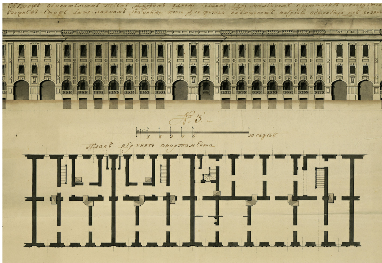
Рис. 2. Чертеж обывательским домам. Архитектор Андрей Меньшой. Ноябрь 1767 года. Фрагмент (фасад и план третьего этажа). [РГИА. Ф. 1293. Оп.166. Астраханская губерния. Д.73]
