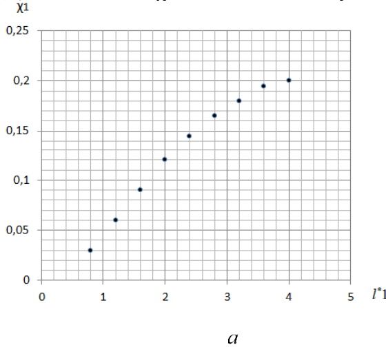
Рис. 2. Изменения удельного распределения ЛФП ( \chi ) при H_{21}^* = const и l_{1i}^* = var для \chi_{1i} — объекта защиты (а) и для \chi_{3i} — молниеприемника СМЗ (б)
