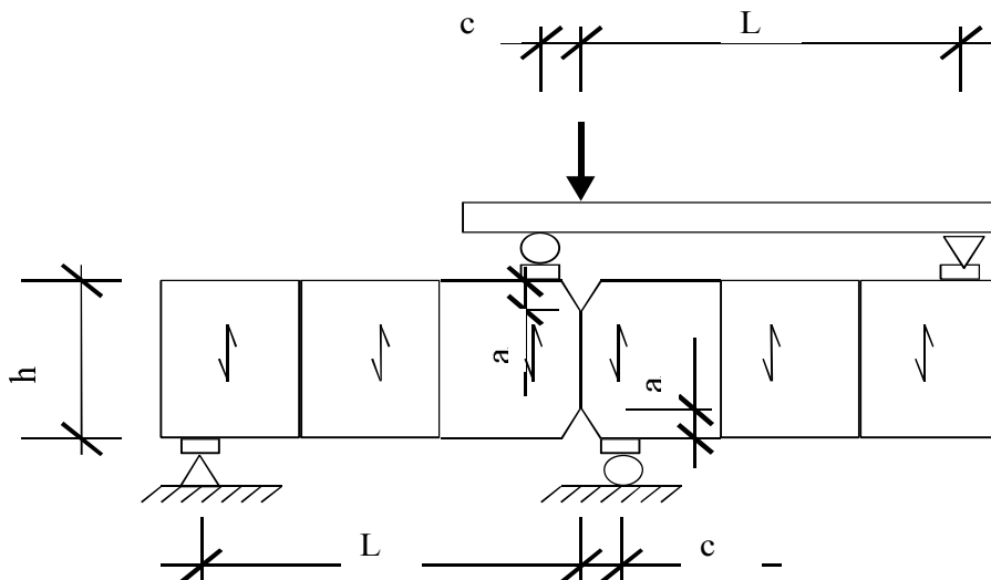
Рис. 1. Призматический образец с двумя поперечными надрезами для определения G_{IIc} .
