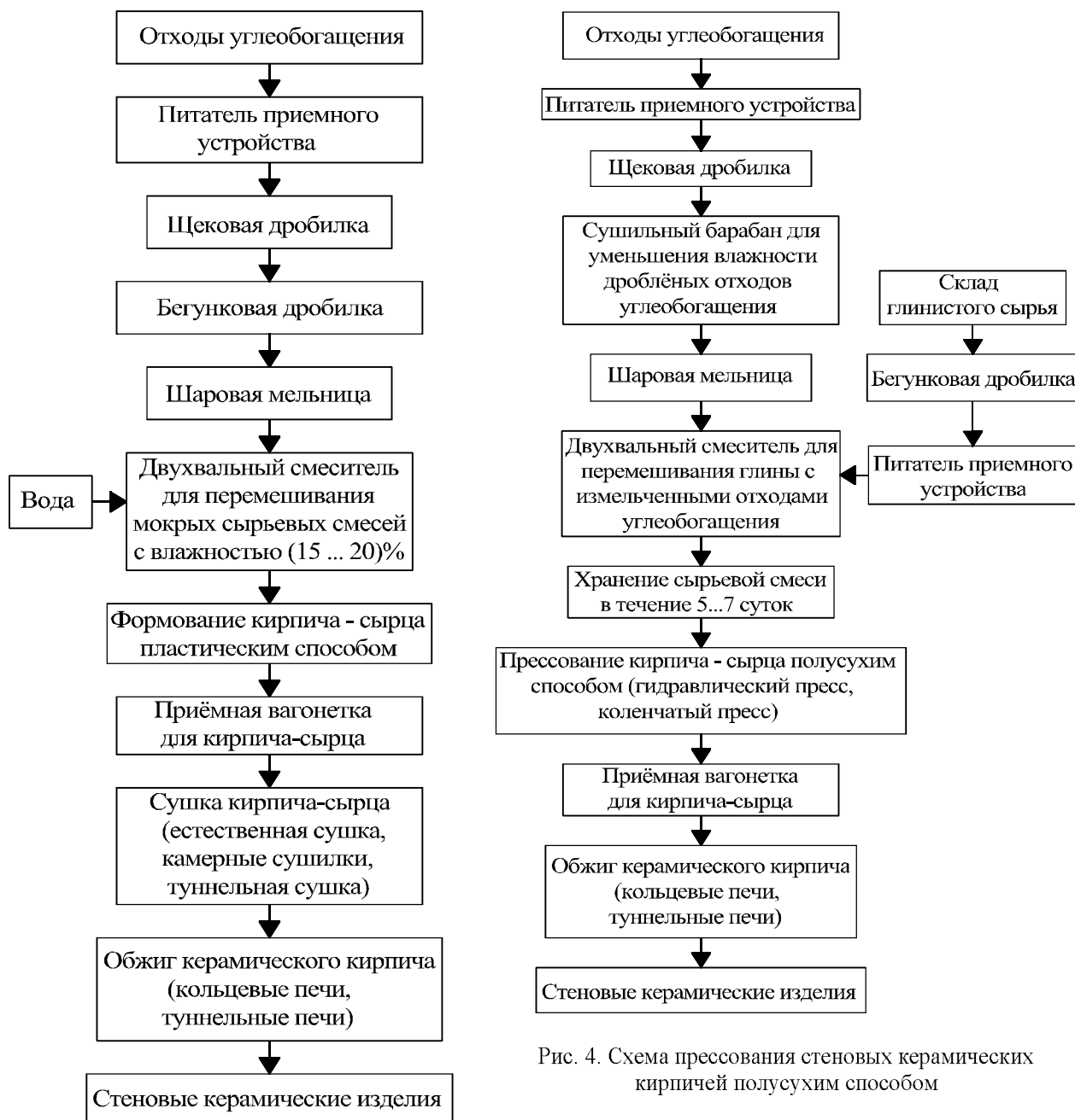
Рис. 3. Схема формирования стеновых керамических кирпичей пластическим способом
