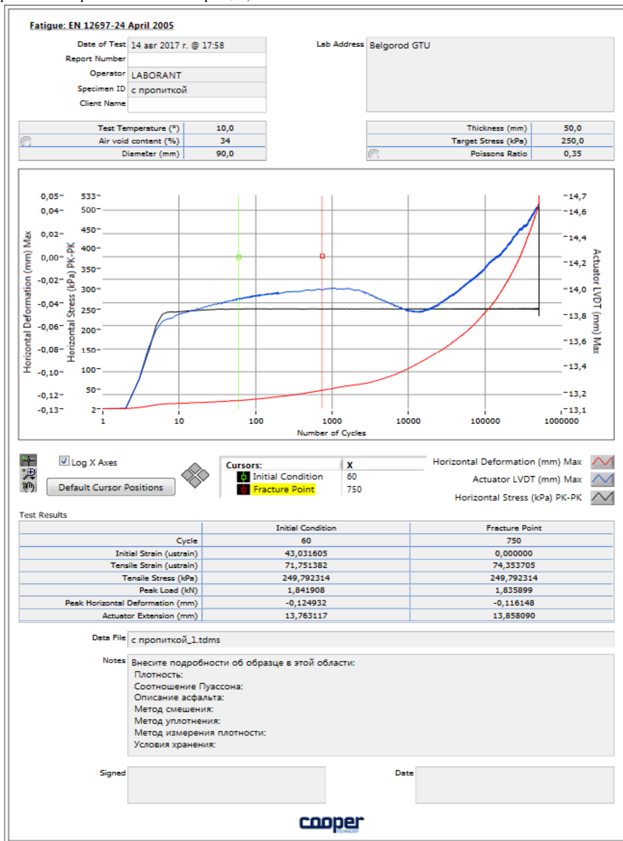
Рис. 1. Показатели усталостной прочности образцов с пропиткой «ДОРЛЮК»
