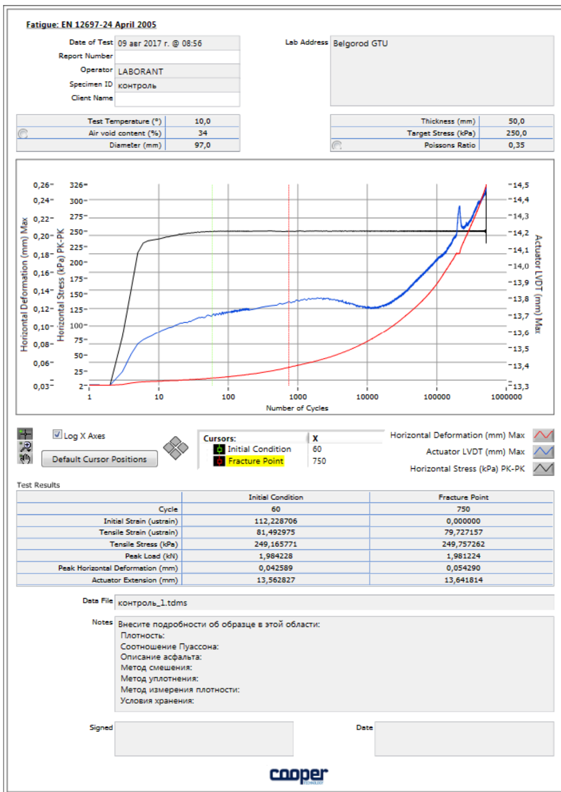
Рис. 2. Показатели усталостной прочности контрольных образцов без пропитки
