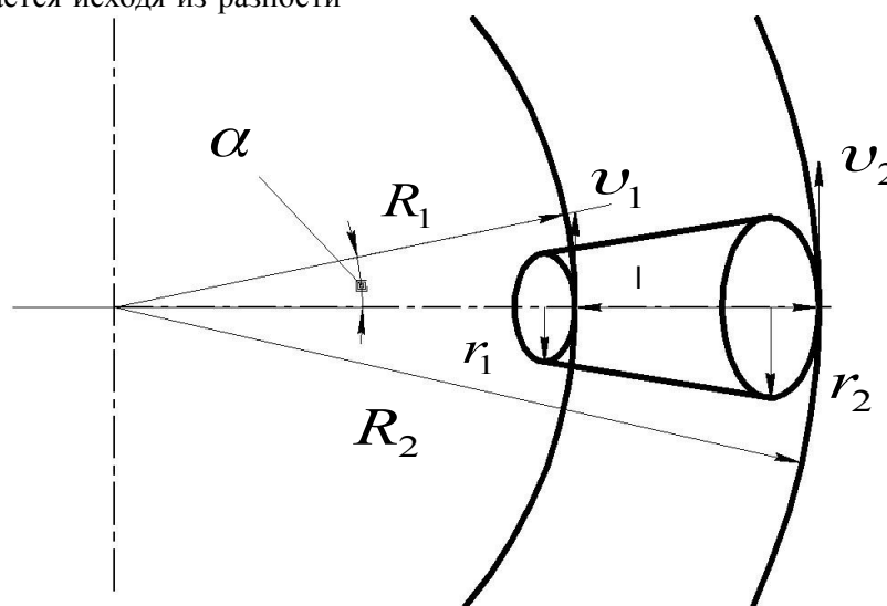
Рис. 4. Распределение линейных скоростей вдоль базовой линии бандажа
