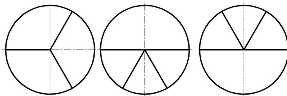
Рис. 7. Варианты схем распределения нагрузки между опорными роликами шестилучевого стэнда при перекосе бандажа
