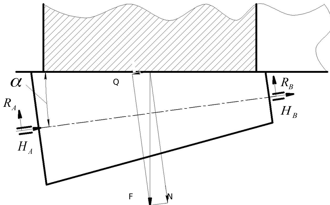
Рис. 6. Схема действия сил на опорный ролик стэнда
