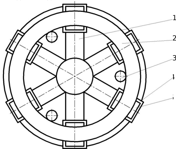
Рис. 2. Концептуальная схема станка:
