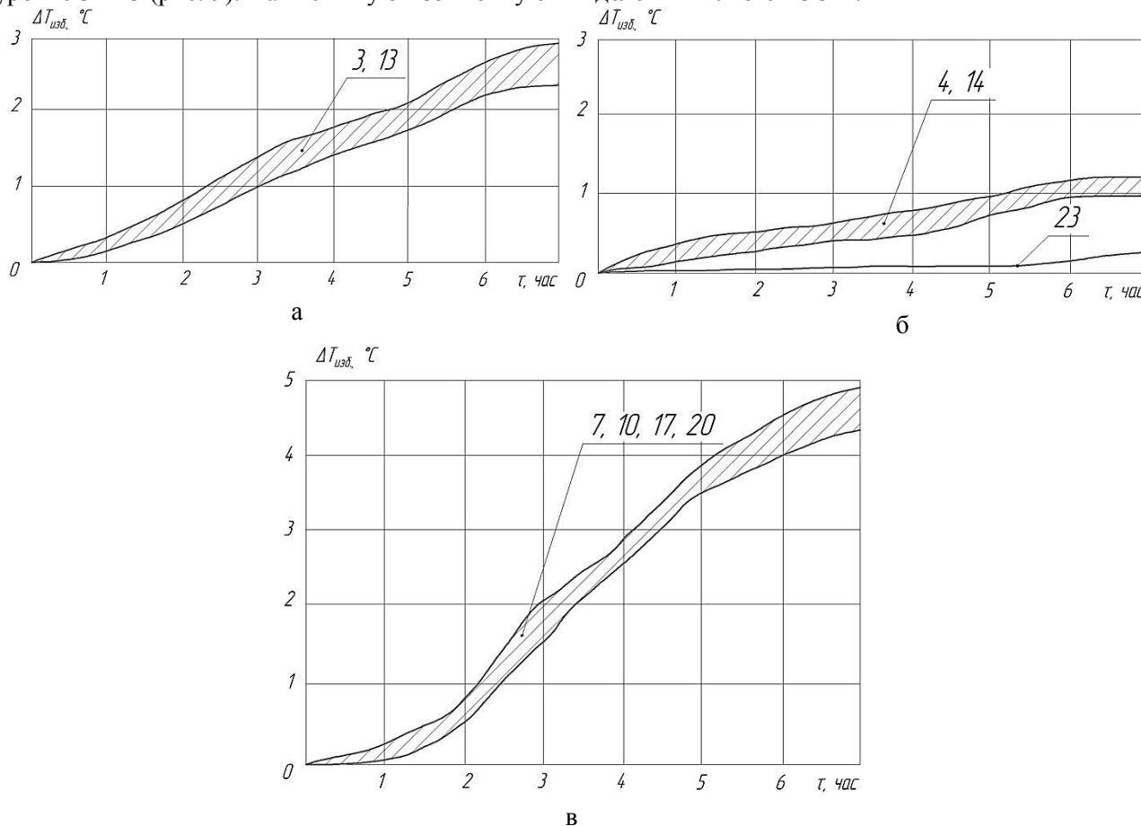
Рис. 8. Изменения температур характерных точек станины станка при работе под тепловой нагрузкой ( N = 6 кВт):
