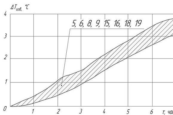
Рис. 7. Изменения температур характерных точек шпиндельной бабки станка при работе под тепловой нагрузкой (N = 6 кВт):
