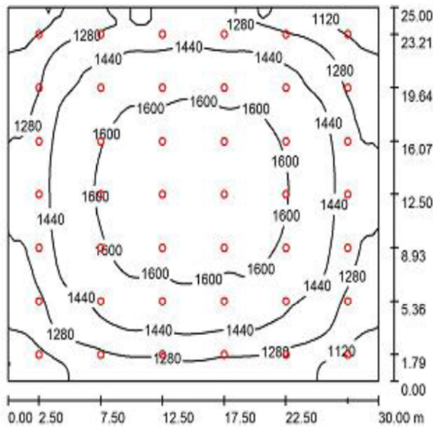
Рис. 2. Величина освещенности и список координат расположения светильников каждой точке арены ДС «Космос»
