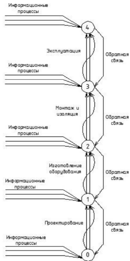
Рис. 3. Системокванты теплотехнической функциональной системы
