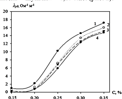
Рис. 1. Концентрационная зависимость удельной электрической проводимости графита в системе гидратационного типа твердения «цементный камень – кварцевый заполнитель – графит» с добавкой 0,05 % (мас.) пластификаторов: 1 – Melflux 2651 F; 2 – Реламикс М2; 3 – ПФМ-НКЛ; 4 – без добавок
