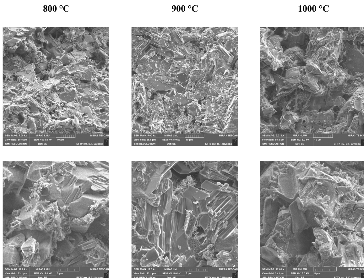
Рис. 3. Морфология новообразований ангидритовых вяжущих в зависимости от температуры обжига
